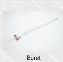
Büret
