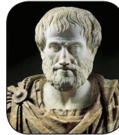
Aristo
