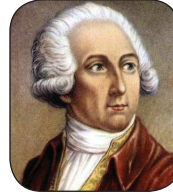
A. Lavoisier
