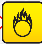
Yakıcı madde
