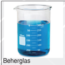
Beherglas
